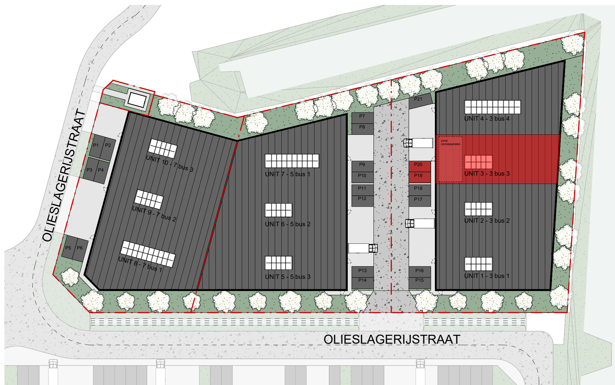
INPLANTINGSPLAN - LIGGING UNIT 3 MET PARKINGS
