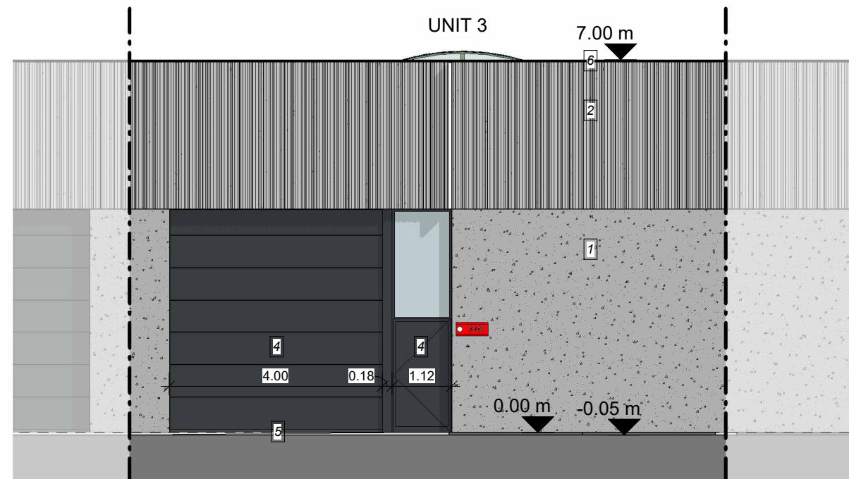
Vorgevel UNIT 3 1 : 100
